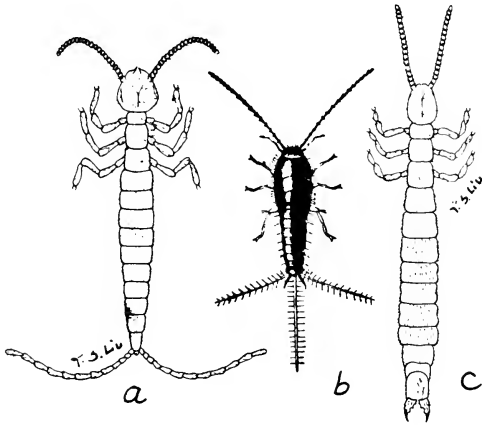
Fig. 49. a, Campodea fragilis Meinert; b, Lepisma sp.; c, Jopyx minemus .
